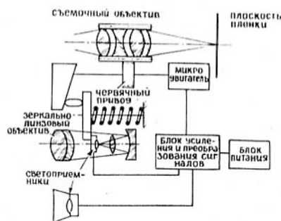
Рис. 5. Схема аппарата «Канон автофокус»
