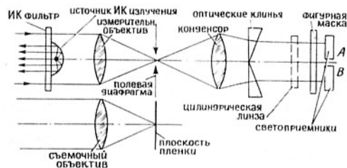
Рис. 2. Двухобъективная система фокусировки
