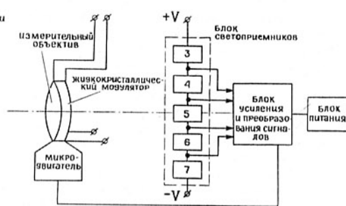
Рис. 6. Схема с модулятором на жидких кристаллах
