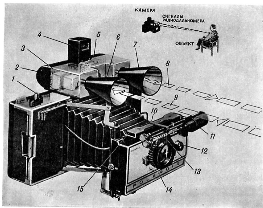
Рис. 1. Автоматическая фокусировка, основанная на принципе локатора: 1 — кнопочный включатель наводки на фокус; 2 — батарея; 3 — преобразователь и другая электронная аппаратура; 4 — видоискатель; 5 — генератор импульсов; 6 — рупорная приемная антенна; 7 — рупорная передающая антенна; 8 — направленные импульсы; 9 — отраженные импульсы; 10 — указатель шкалы наводки; 11 — микродвигатель; 12 — фотоэлемент автоматического экспонометра; 13 — червячный привод наводки на фокус; 14 — кольцо фокусировки; 15 — переменное сопротивление системы обратной связи
