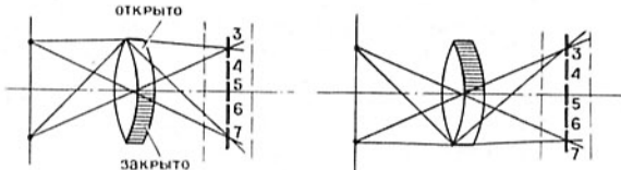
Рис. 7. Ход лучей на светоприемники
