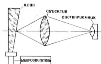
Рис. 4. Система с вращающимся клином
